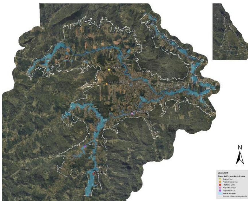
Figura 67 – Obras de Drenagem e áreas de inundação em São João do Itaperiú.
